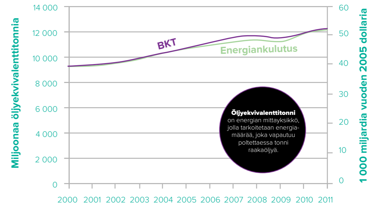
KUVAAJA 6 Maailman energiankulutus ja BKT vuosina 2000–2011
